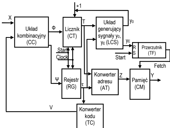
Rys. 2. Mikroprogramowany układ sterujący CMCU_EM
