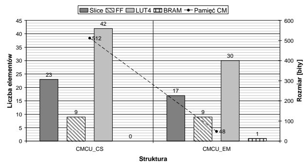
Rys. 3. Zużycie zasobów sprzętowych dla sieci testowej we_00 (area level 1)
