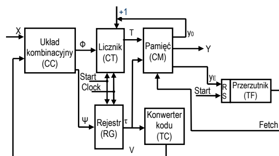
Rys. 1. Mikroprogramowany układ sterujący CMCU_CS
