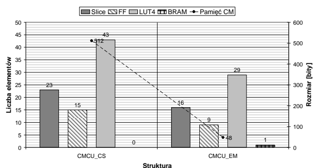
Rys. 6. Zużycie zasobów sprzętowych dla sieci testowej we_00 (□el□□ level 2)
