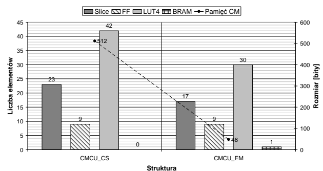
Rys. 4. Zużycie zasobów sprzętowych dla sieci testowej we_00 (area level 2)
