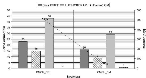
Rys. 5. Zużycie zasobów sprzętowych dla sieci testowej we_00 (□el□□ level 1)
